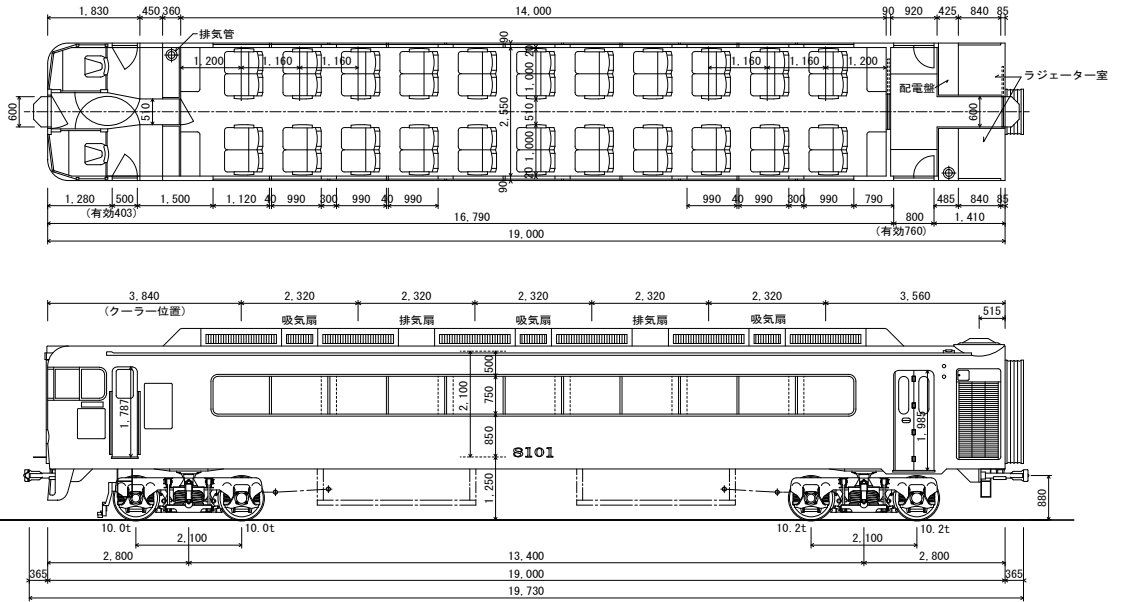
名鉄8100型 1等車 DCG 座席定員 44人
