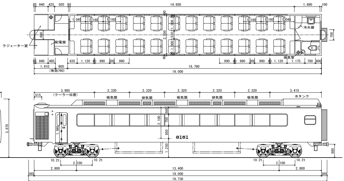
名鉄8150型 1等車 D1 座席定員 48人
