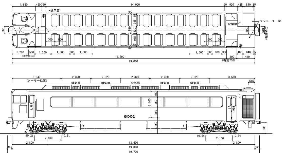
名鉄8000型 2等車 DCG 座席定員 60人
