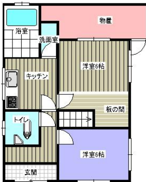
1階 平面図
