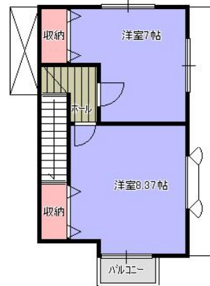
2階 平面図
