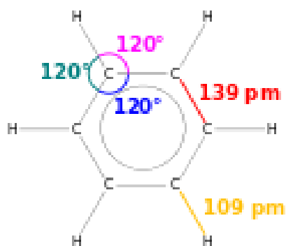
Fig. 11 Benzene molecule
