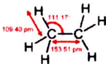
Fig. 9 Ethane molecule
